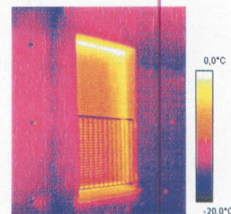
Termografski posnetek okna na nizkoenergijski hiši, ki predstavlja toplotni most v ovojni zgradbi. Okno z dvoslojno zasteklivitvijo in okvirjem, ki ni toplotno izoliran ( U_w = 0,95 \text{ W}/(\text{m}^2\text{K}) ), je vgrajeno na zunanji rob zidane stene, izolirane z 20 cm toplotne izolacije. Okno in izvedba nista primerna za pasivno hišo.
