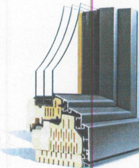
Okenski okvir iz lesa – toplotna prehodnost skozi okvir je zmanjšana z zaprtimi komorami zraka (Foto: arhiv M Sora)
