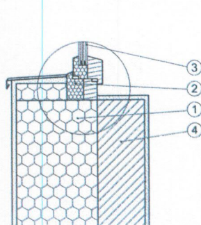
Zrakotesna vgradnja okna v masivno steno
