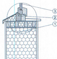
Zrakotesna vgradnja okna v lahko steno
