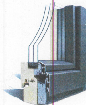
Okenski okvirji za pasivne hiše – dodatna plast toplotne izolacije izboljša toplotno izolativnost (foto: zgoraj arhiv Internorm, spodaj arhiv M Sora)
