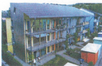
V pasivni hiši so okenske površine večje, saj omogočajo dobitke sončnega sevanja.
