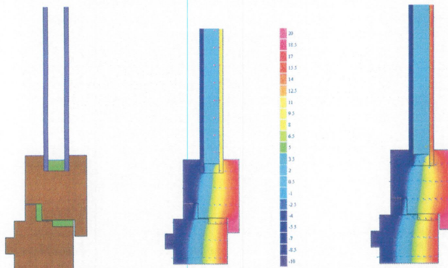
Temperaturni profil prečnega prereza okna z dvojno zasteklivitvijo in lesenim okvirjem z dvakratnim tesnjenjem; sredina: starejša dvojna »termopan« zasteklitev ( U > 2,5 \text{ W}/(\text{m}^2\text{K}) ); desno: zasteklitev s stekli z nizkoemisijским nanosom, medstekelni prostor je polnjen s plinom argonom ( U \approx 1,2 \text{ W}/(\text{m}^2\text{K}) ) (izračun in risba: Miha Praznik)
