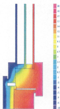
Temperaturni profil prečnega prereza okna s trislojno zasteklivitvijo z dvema nizkoemisijским nanosoma in plinom argonom v medstekelnem prostoru ( U \approx 0,7\text{--}0,8 \text{ W}/(\text{m}^2\text{K}) ) (izračun in risba: Miha Praznik)
