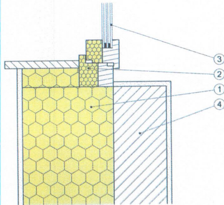
Pravilna vgradnja okna v masivno in lahko leseno steno
